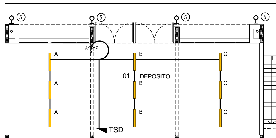
PLANTA NIVEL - 2,80
