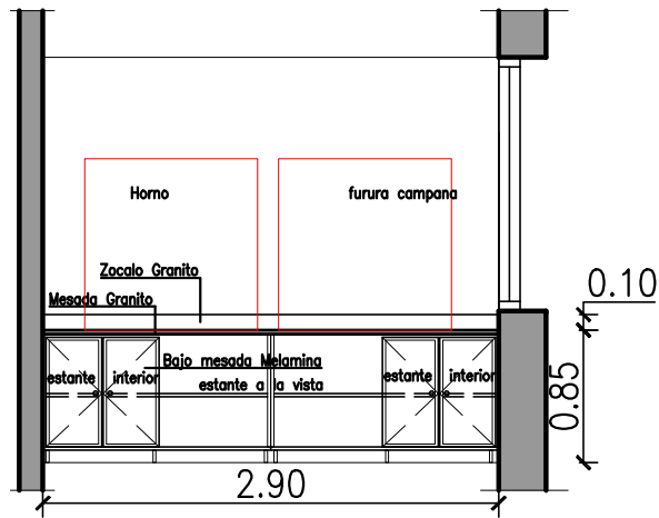
VISTA A-A
