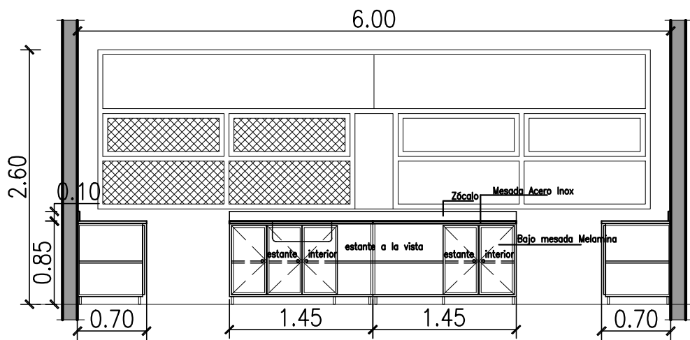
VISTA B-B
