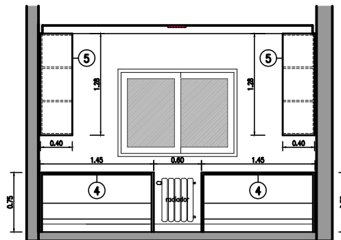
CORTE VISTA 3-3
