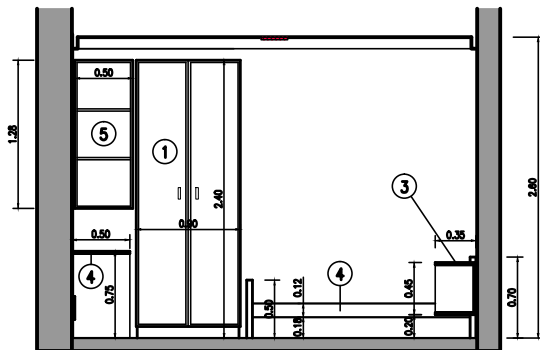
CORTE VISTA 1-1
