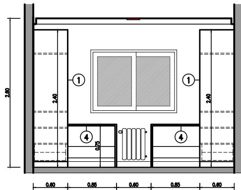
CORTE VISTA 2-2
