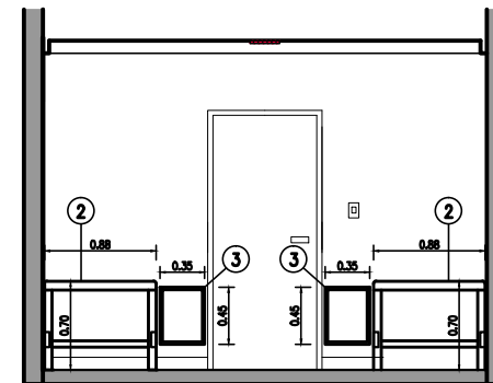
CORTE VISTA 4-4
