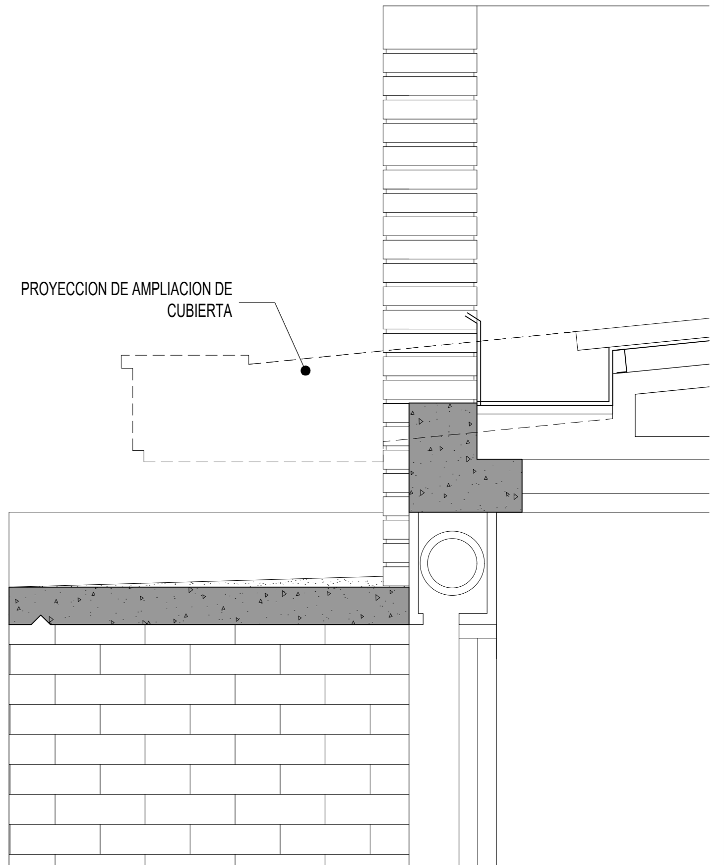
CORTE A-A // ESTADO ACTUAL
