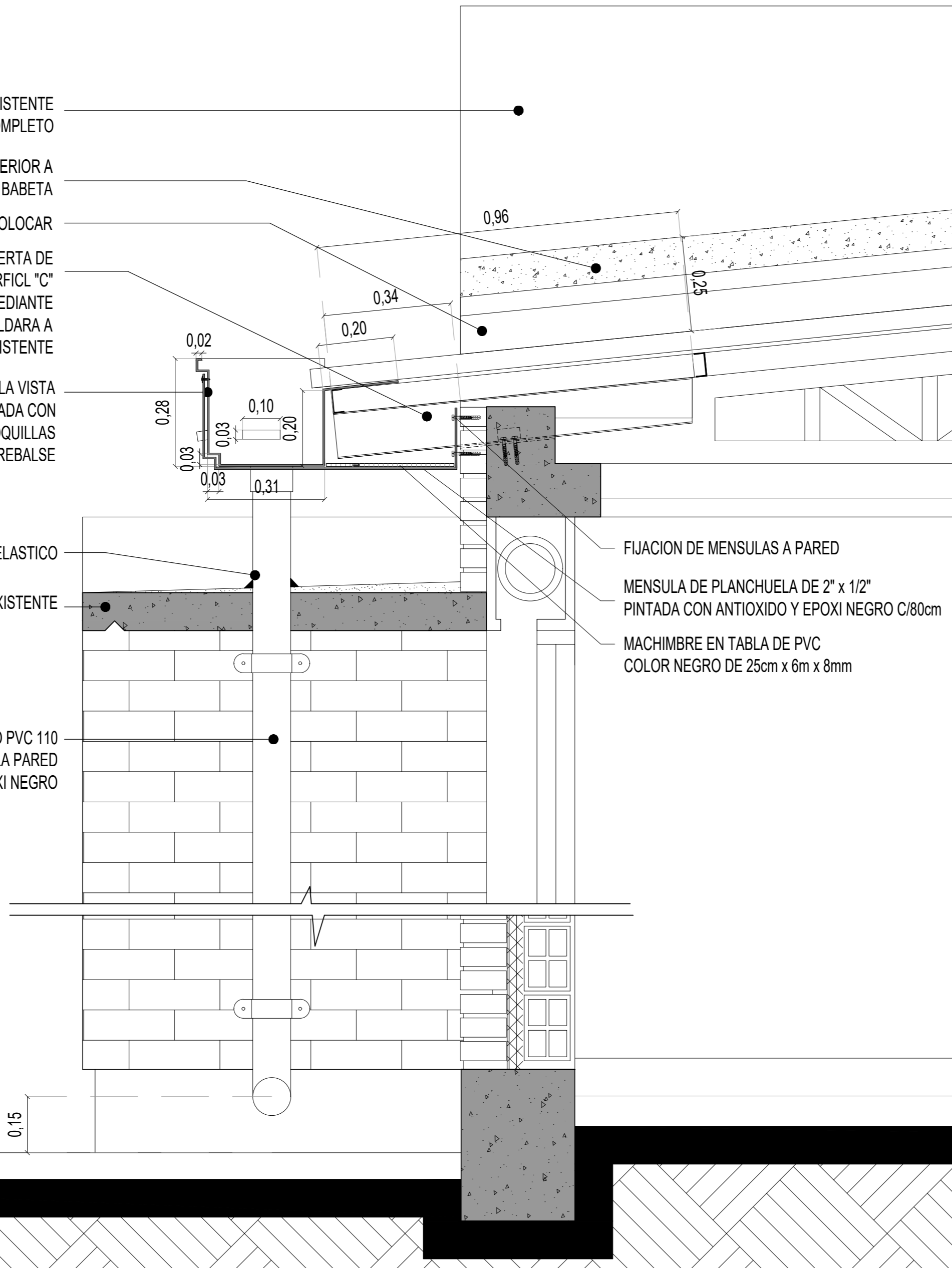
CORTE A-A // ESTADO MODIFICADO
