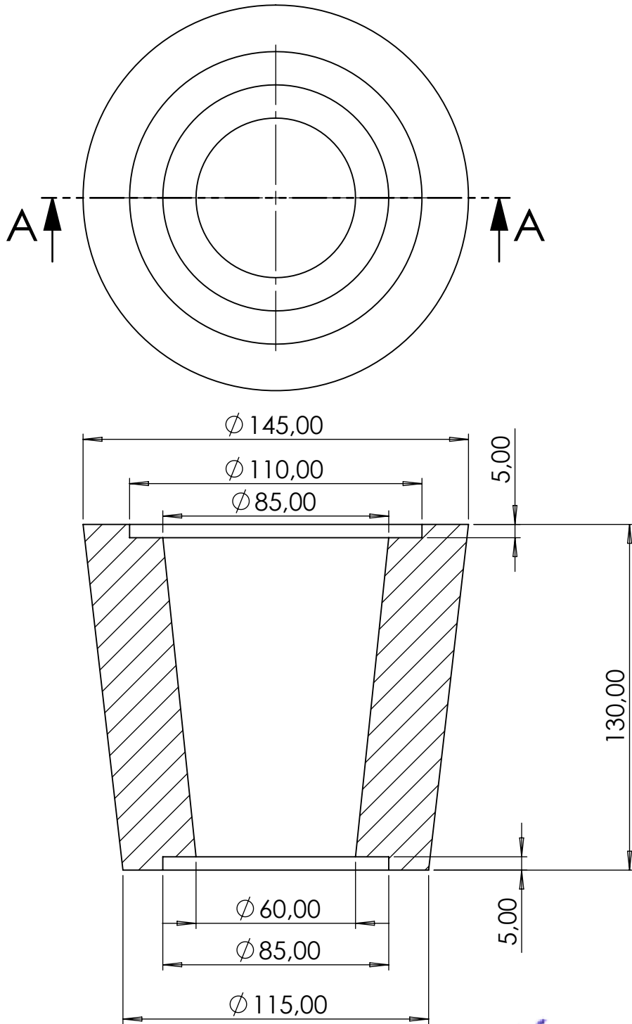
SECCIÓN A-A ESCALA 1 : 2
