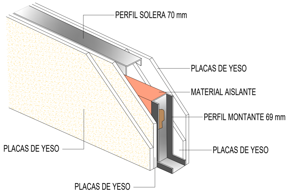
DETALLE TABIQUE DOBLE PLACA DE YESO
