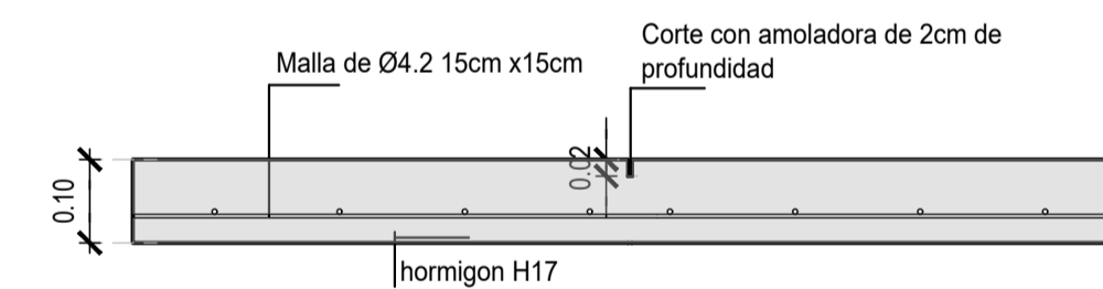
DETALLE JUNTA DILATAZION
