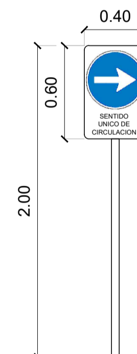
CARTEL SENTIDO CIRCULACION
