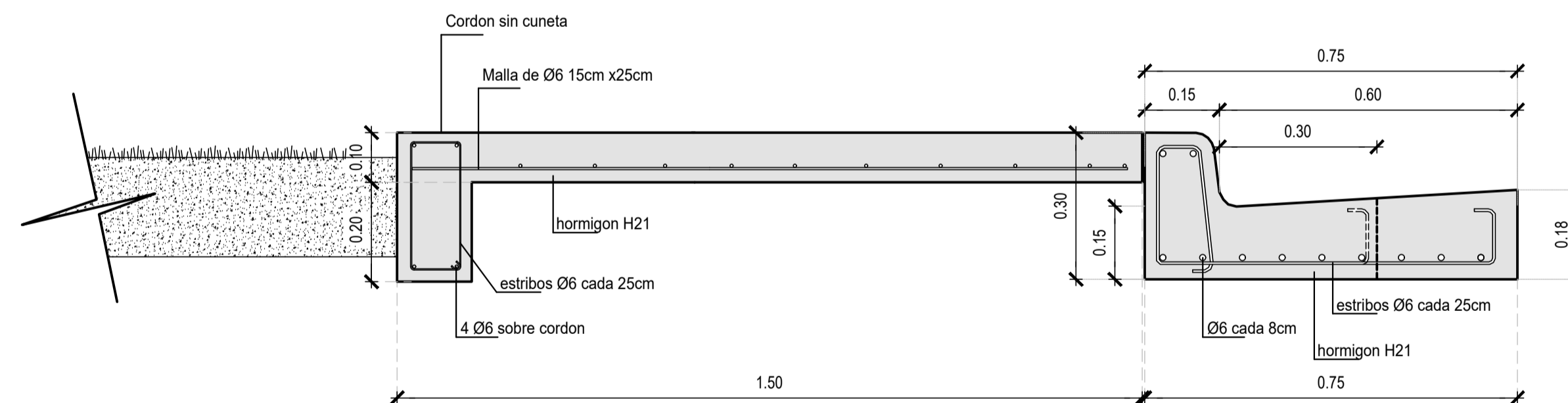
DETALLE VEREDA CON CORDON CUNETA
