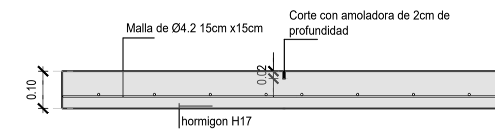
DETALLE JUNTA DILATAZION
