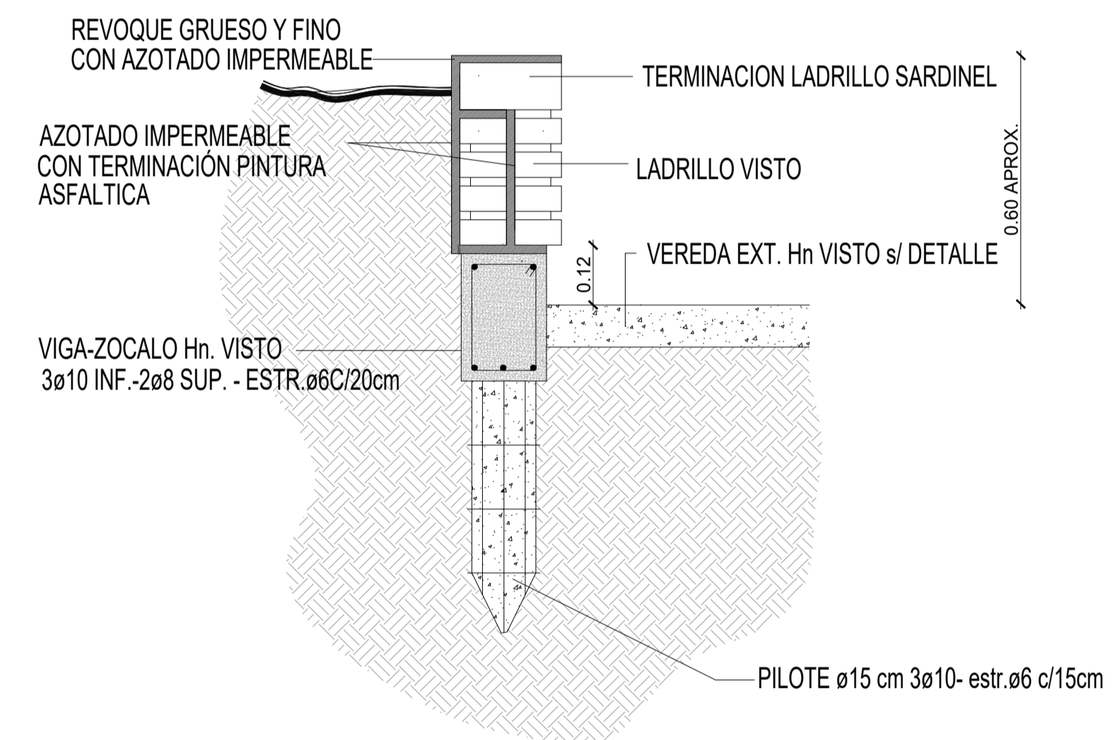
DETALLE MURO DE CONTENCIÓN ESCALA= 1:12,5
