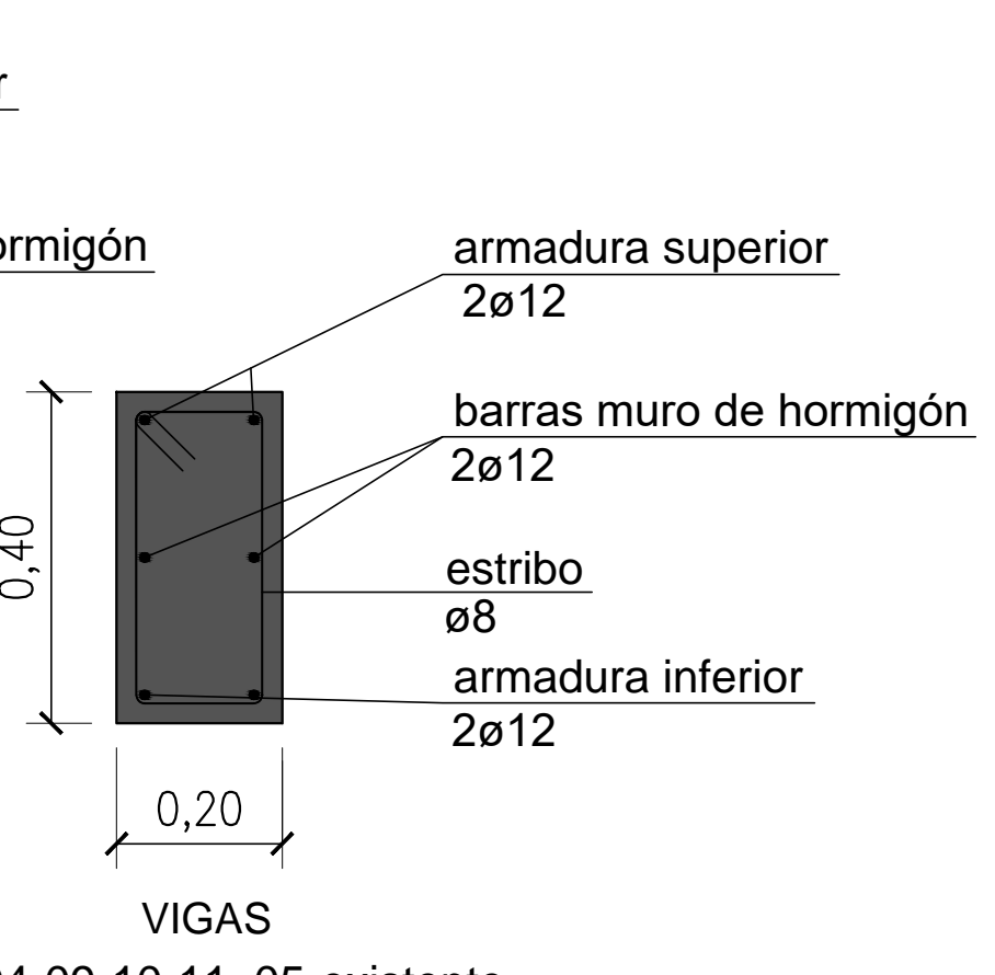
VIGAS SOBRE EDIFICIO EXISTENTE
