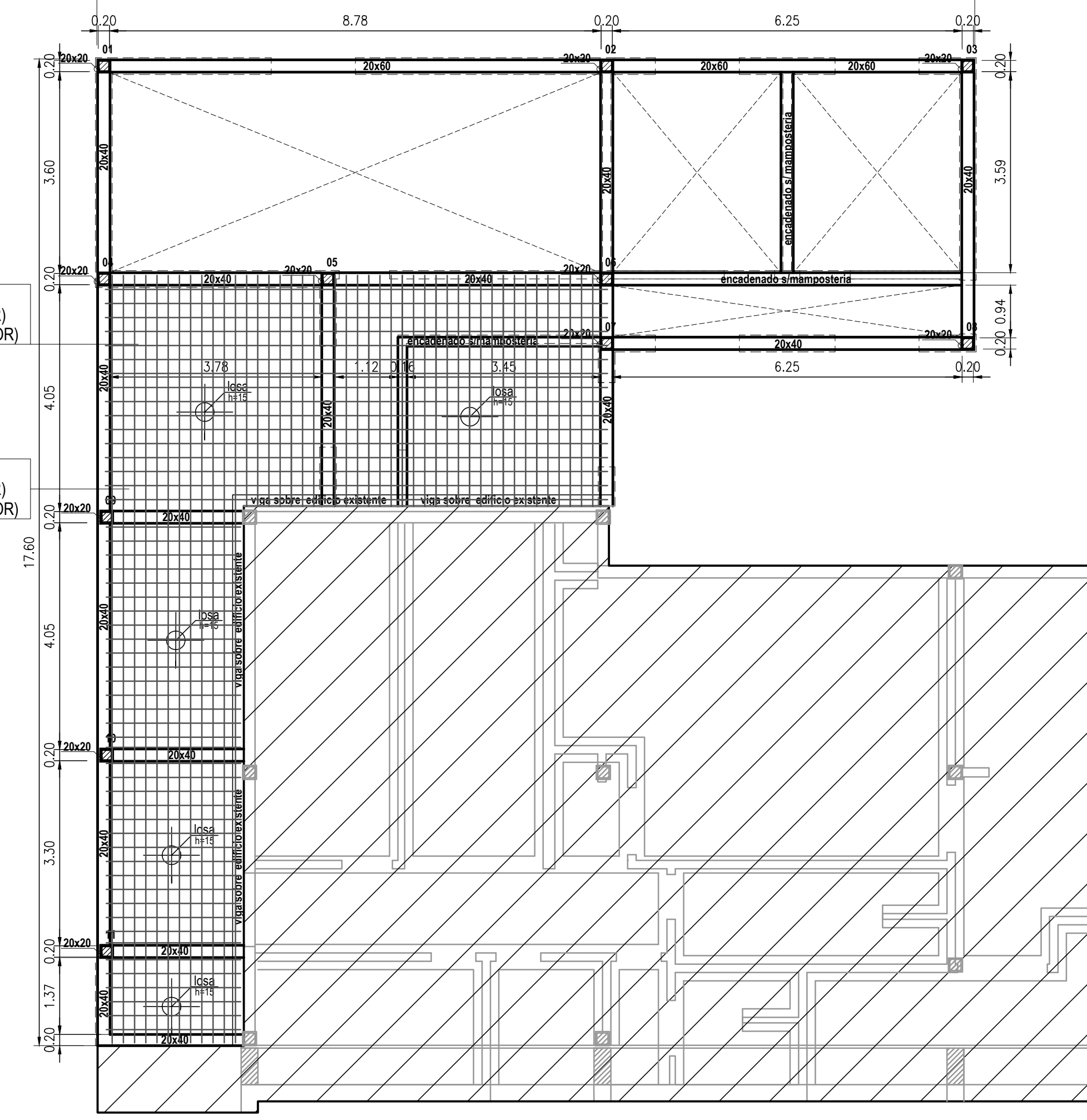
LOSAS Y VIGAS DE ENCADENADO
