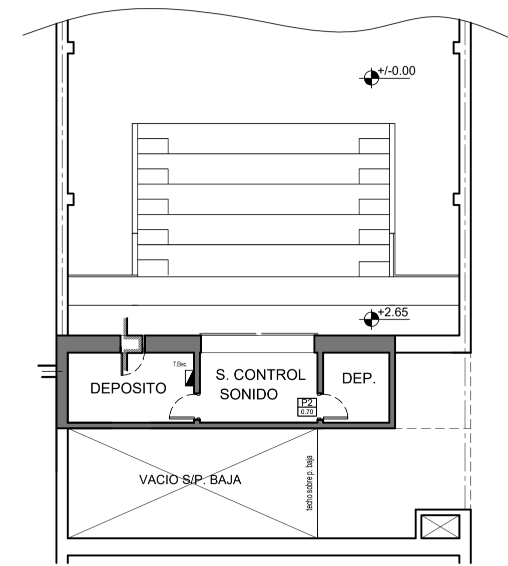
PLANTA S/TRIBUNA
