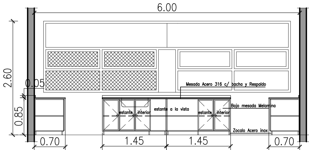
VISTA B-B
