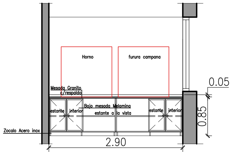
VISTA A-A
