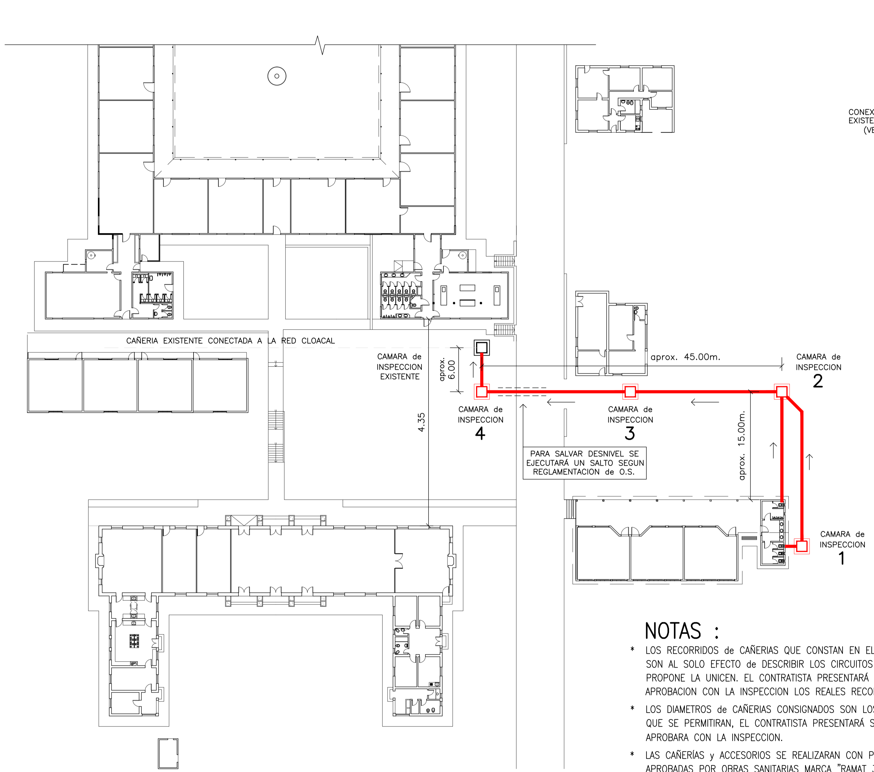
ESQUEMA GENERAL de CONEXIÓN
