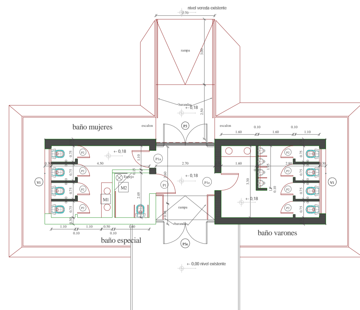
PLANTA REDISEÑADA
