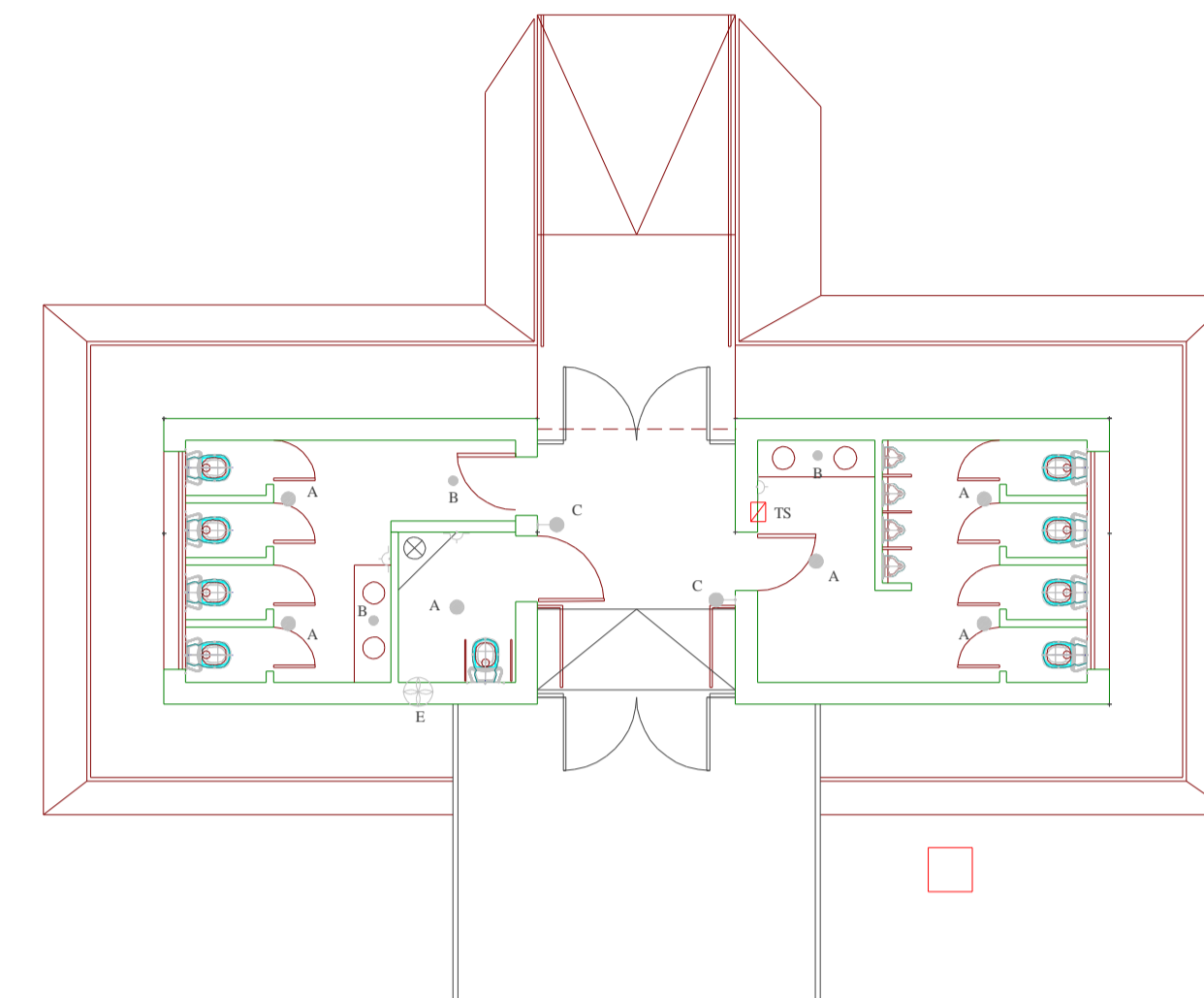
ESQUEMA ELECTRICO
