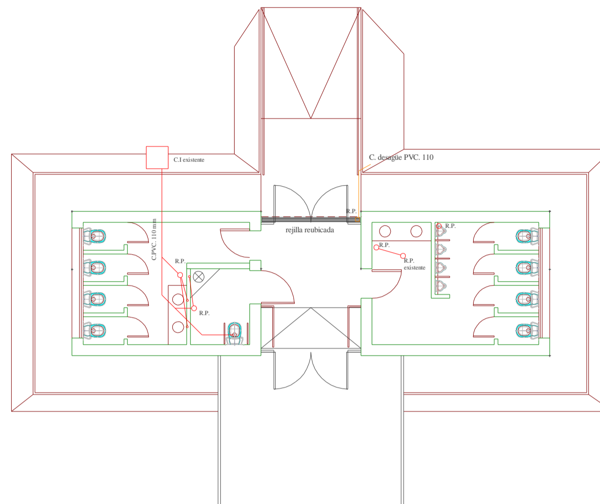
ESQUEMA CLOACAL
