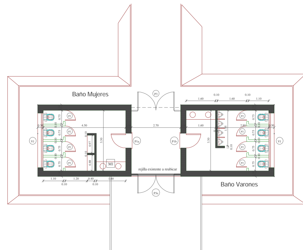
PLANTA EXISTENTE
