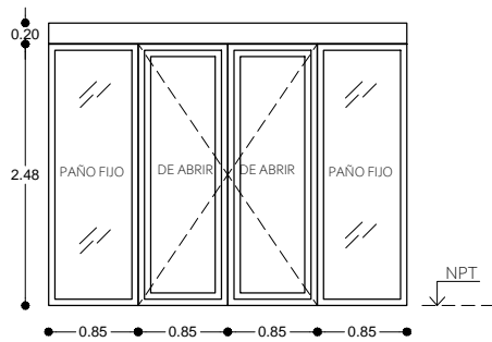
VISTA (P1)
