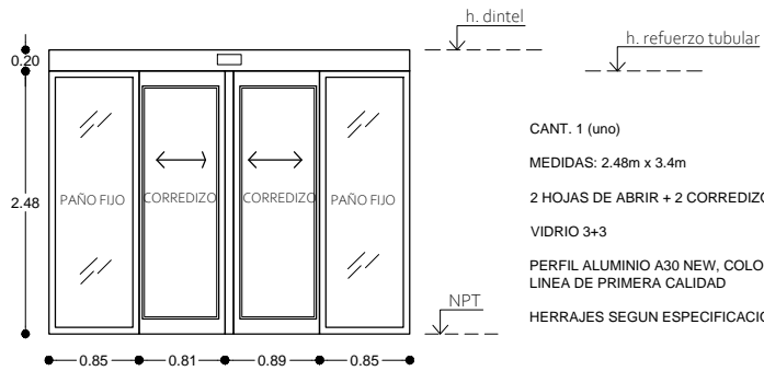
VISTA (P2)
