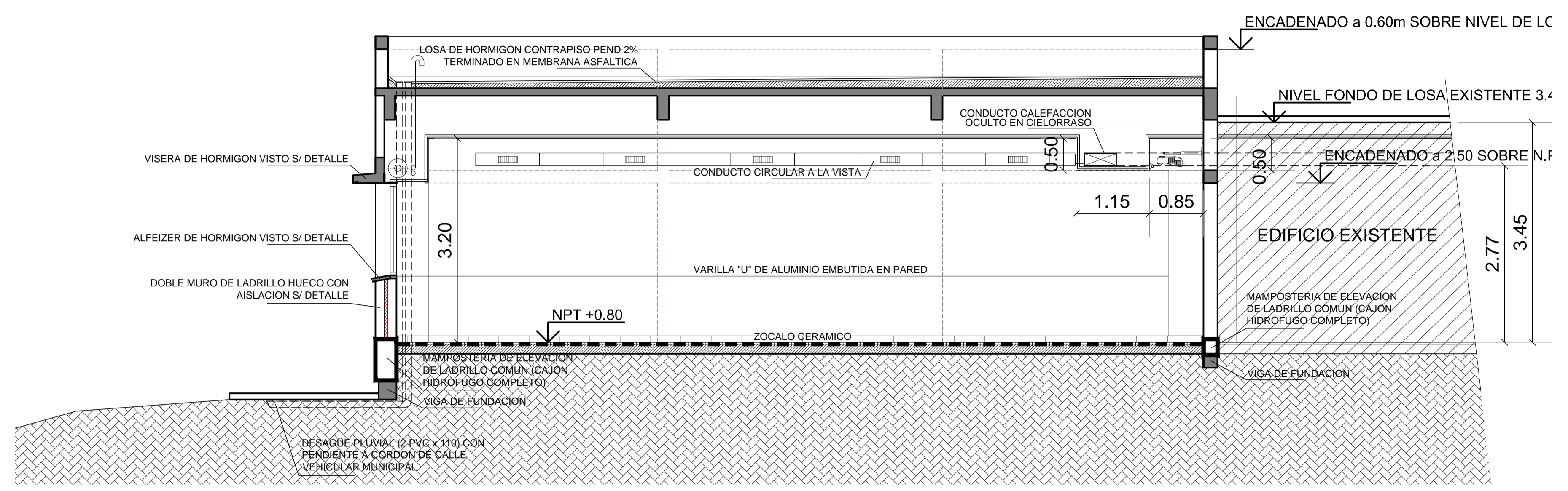
CORTE A-A
