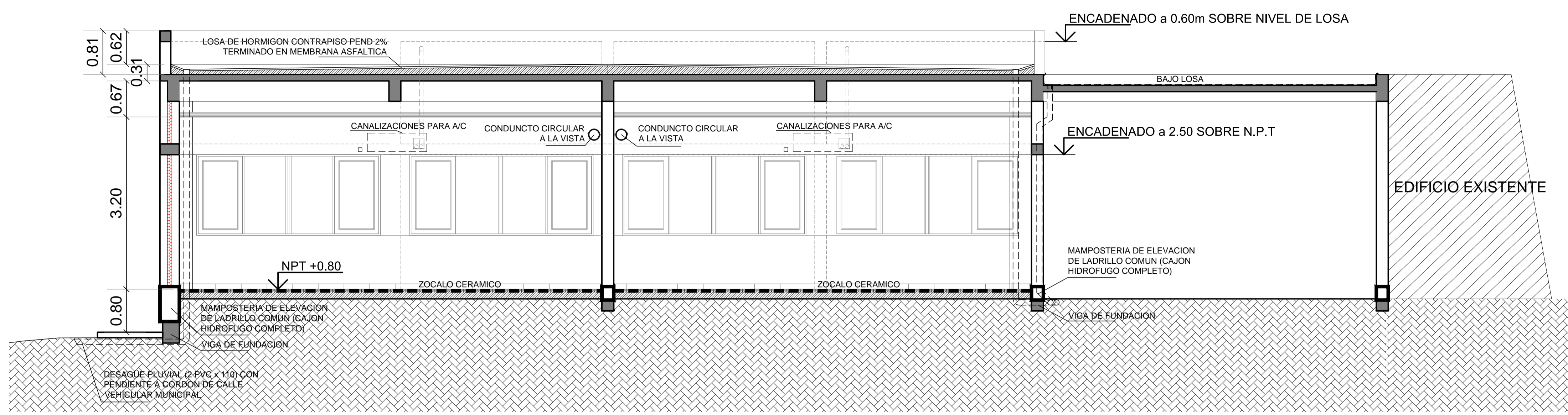
CORTE B-B
