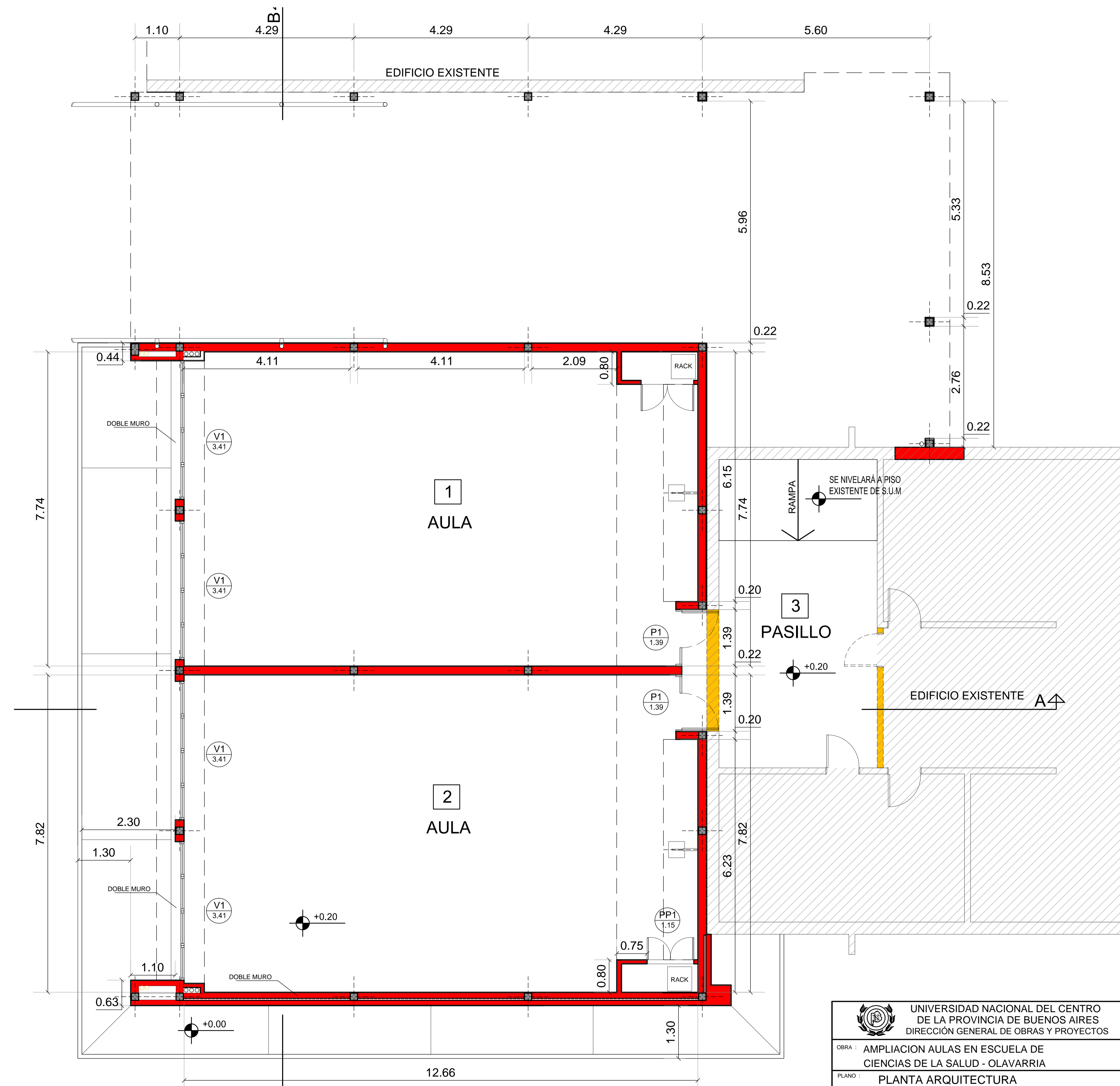
PLANTA BAJA
