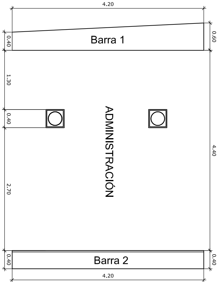
ADMINISTRACIÓN - BARRA PLANTA
