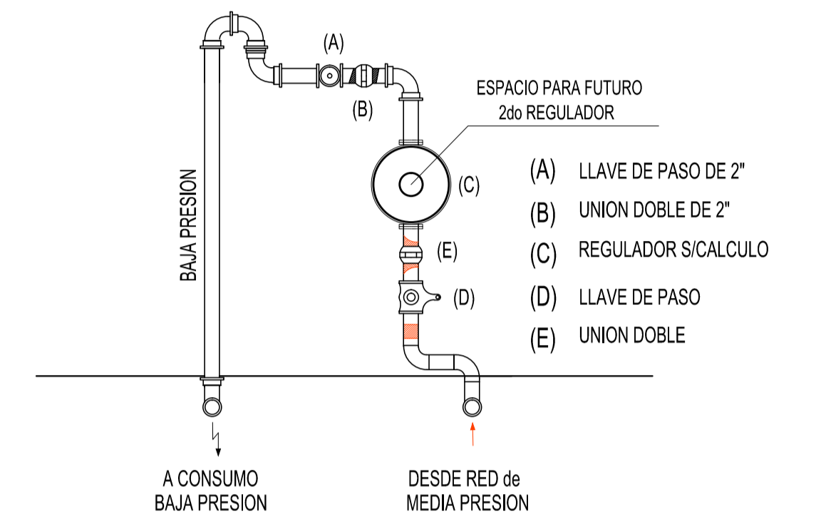
VISTA EQUIPO DE REGULACION
