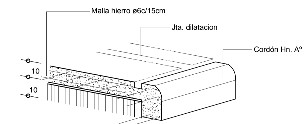
DETALLE JUNTA DE DILATACION (colocada cada 3 mts.) Y CORDON VEREDA
