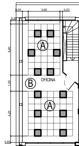
PLANTA ALTA
