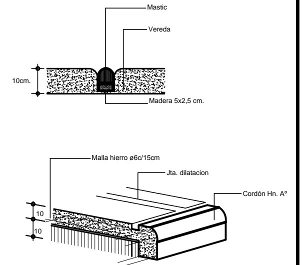
DETALLE JUNTA DE DILATACION (colocada cada 3 mts.) Y CORDON VEREDA
