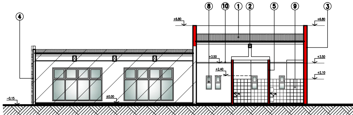
CORTE A-A'
