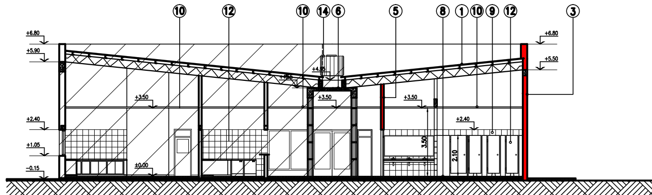
CORTE B-B'
