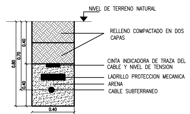
DETALLE TENDIDO SUBTERRANEO
