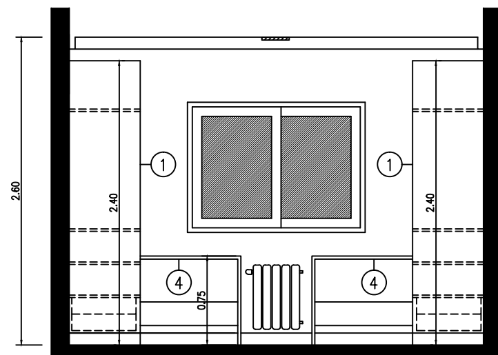
CORTE VISTA 2-2
