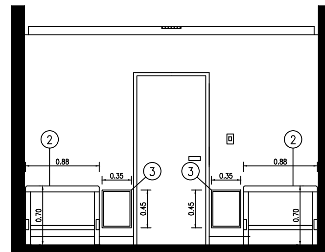
CORTE VISTA 4-4
