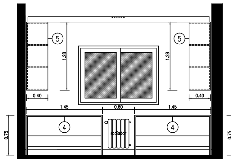
CORTE VISTA 3-3
