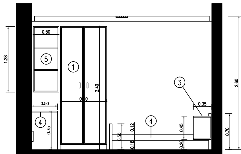
CORTE VISTA 1-1
