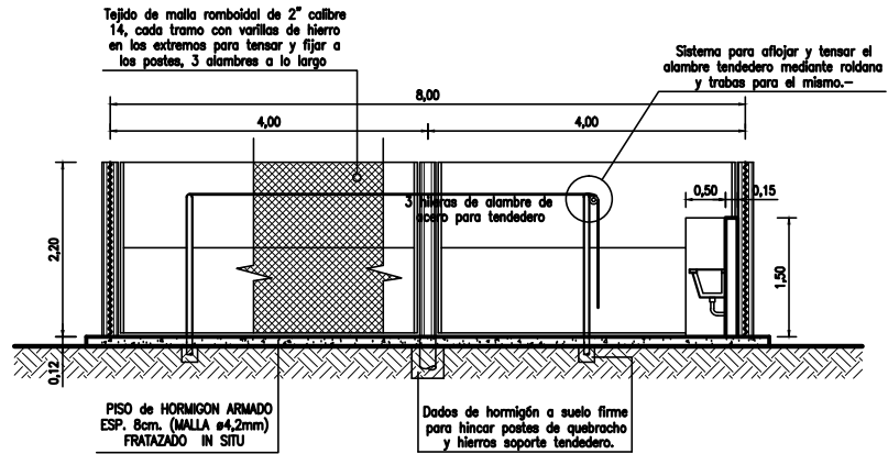
CORTE A-A'
