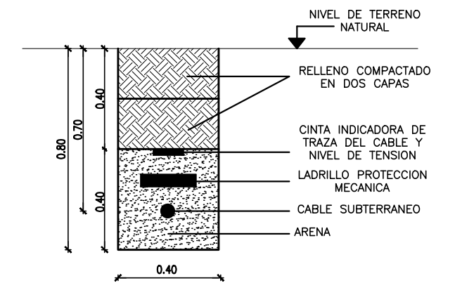
DETALLE TENDIDO SUBTERRANEO
