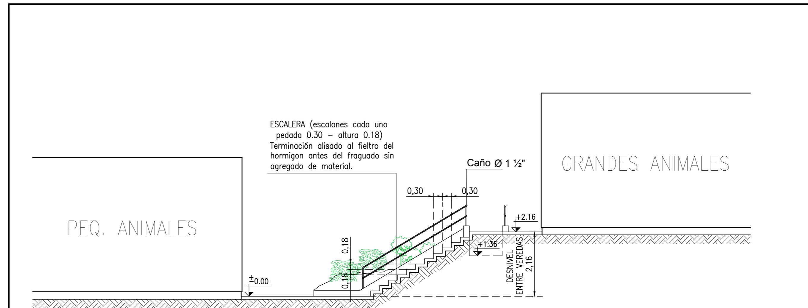
CORTE A-A'
