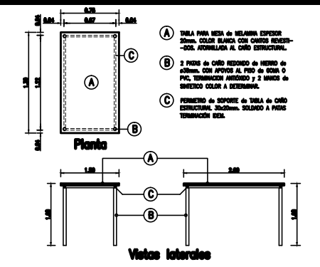
DETALLE de MESAS COMEDOR 12 (CANT. 5)
