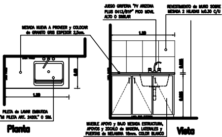
DETALLE MESADA 11 (CANT. 1)
