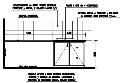
DETALLE MESADAS 12 y 13 - VISTA (CANT. 1)
