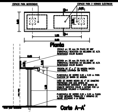
DETALLE de BARRA APOYO 10 (CANT.1)
