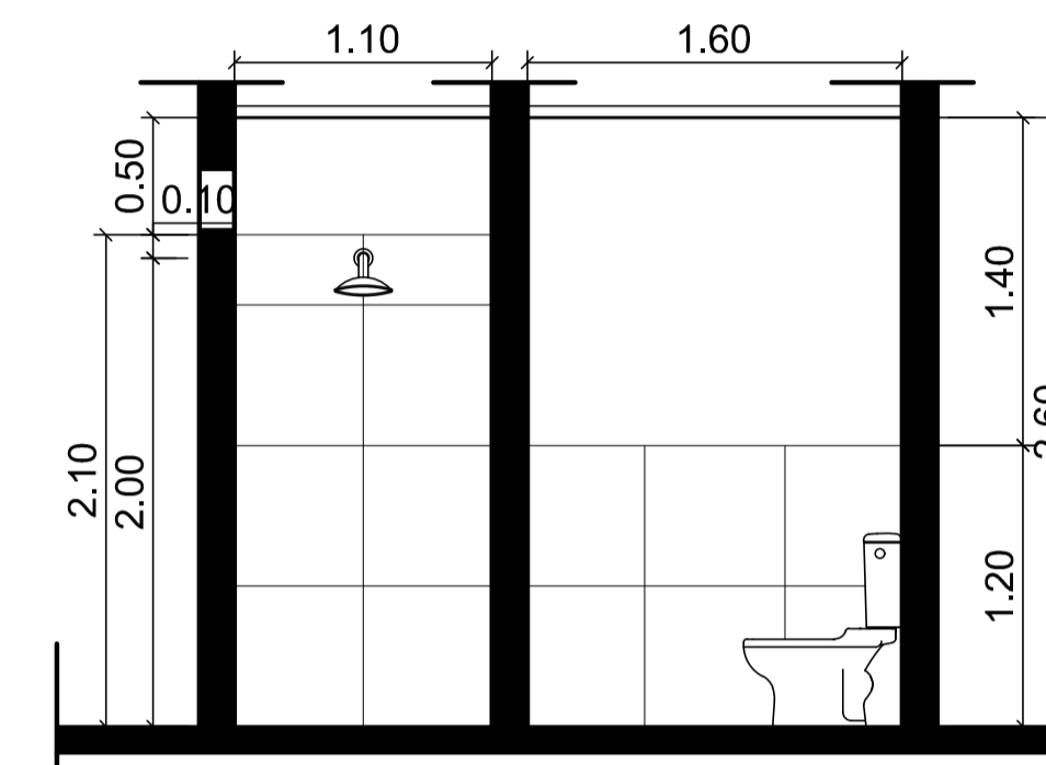
CORTE VISTA 5-5
