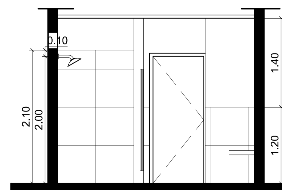
CORTE VISTA 4-4
