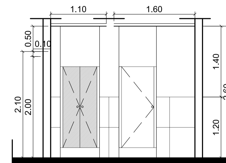
CORTE VISTA 6-6
