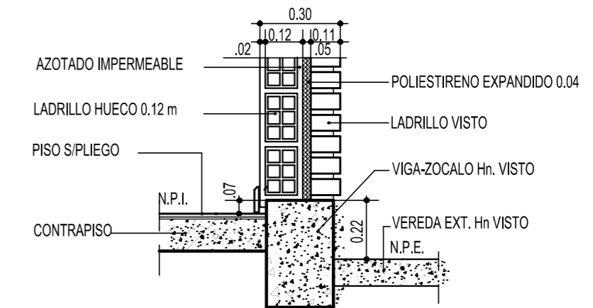
DETALLE MURO EXTERIOR
