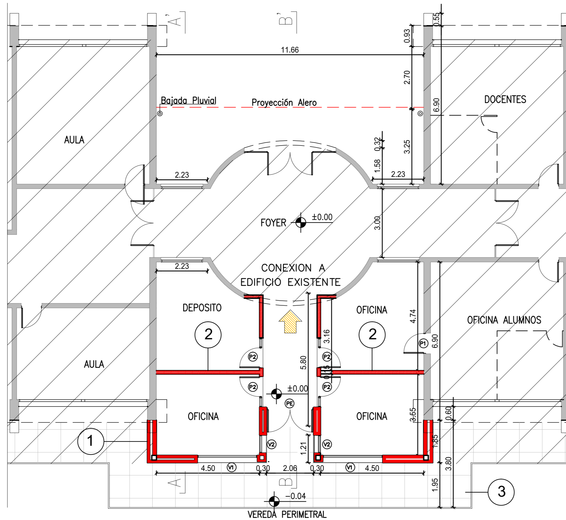
PLANTA GENERAL SUPERFICIE A AMPLIAR: 93,00m 2
