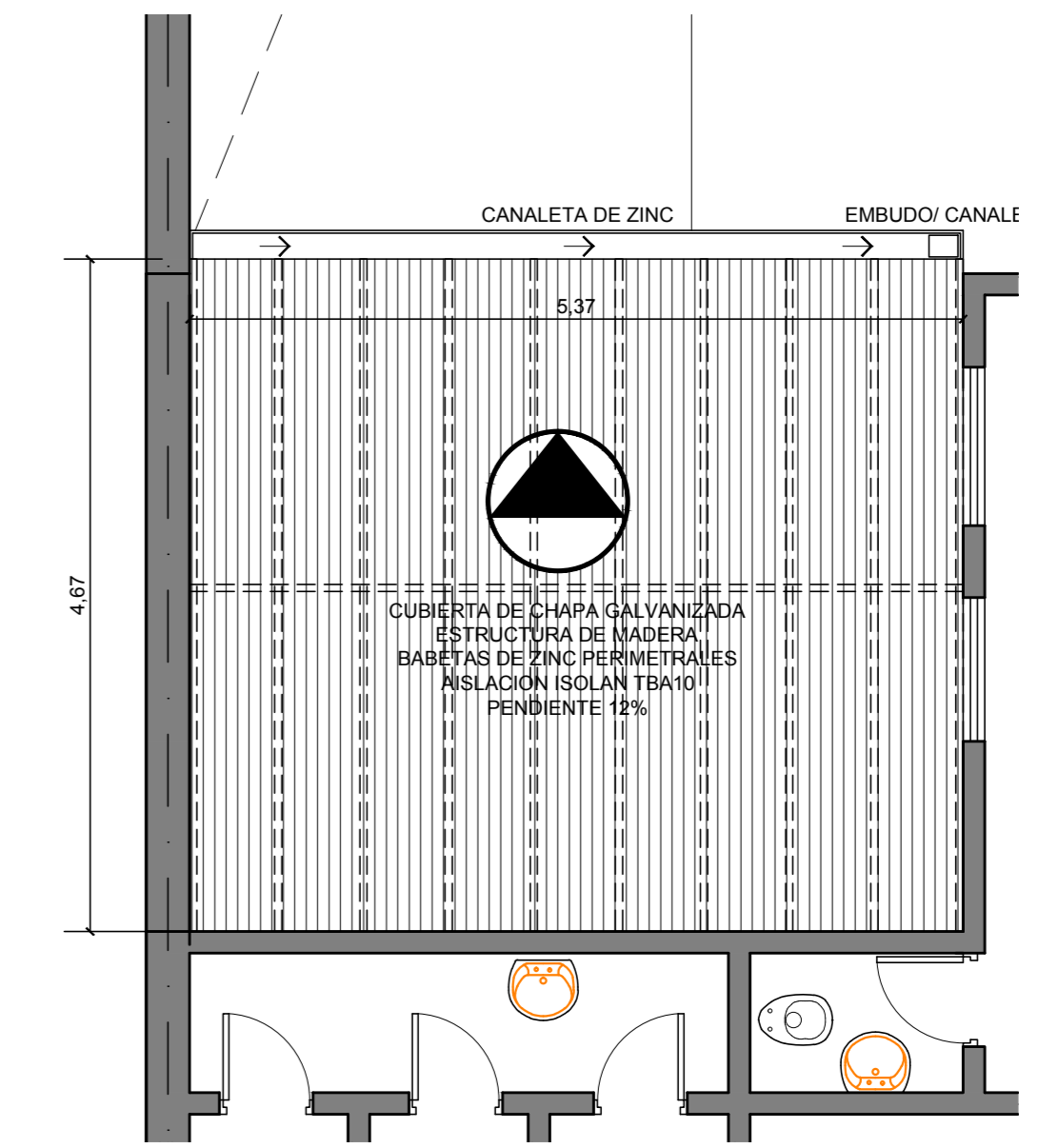
PLANTA DE TECHO
