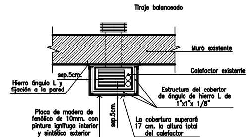
DETALLE COBERTURA de CALEFACTORES
