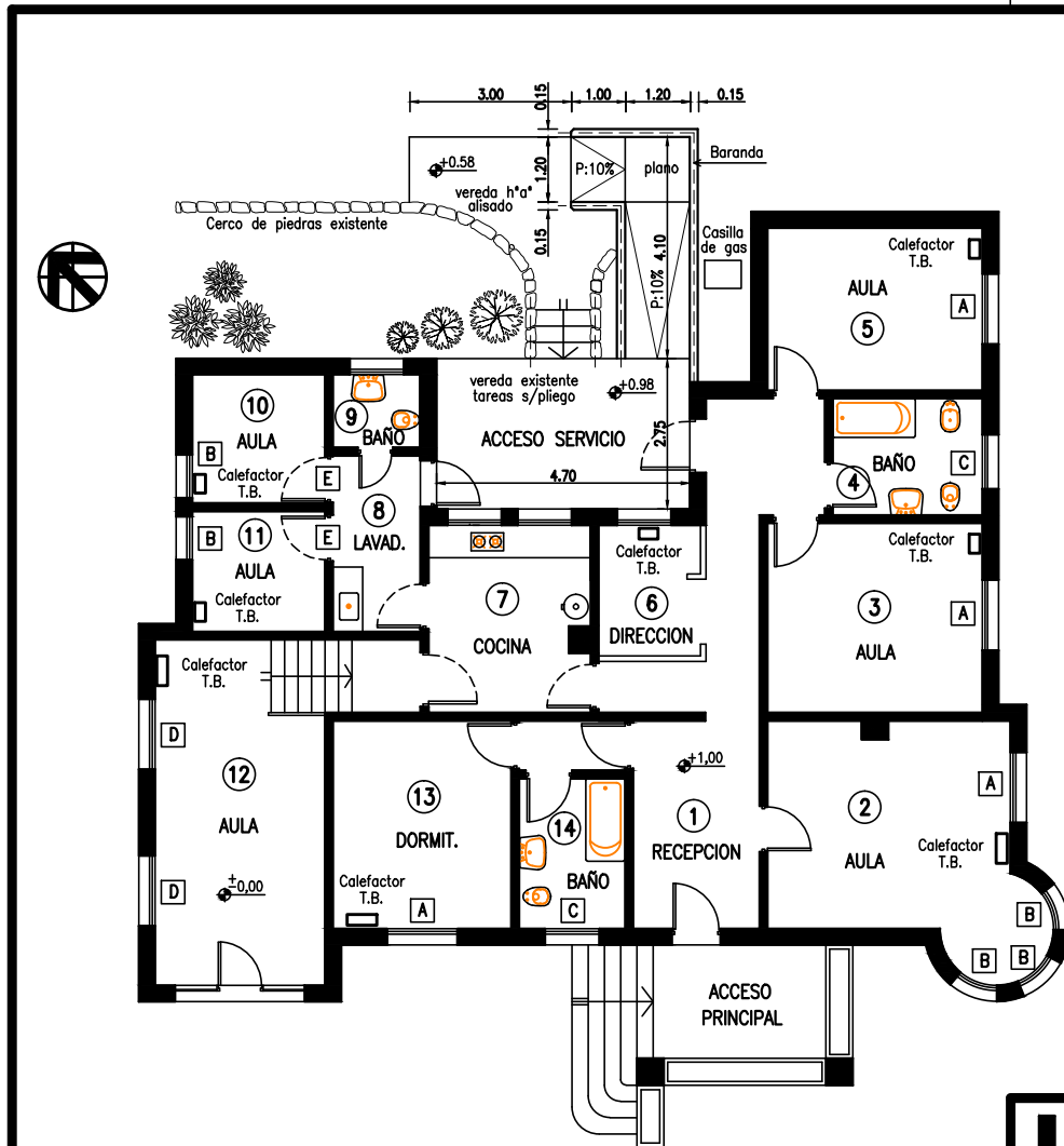
PLANTA GENERAL
