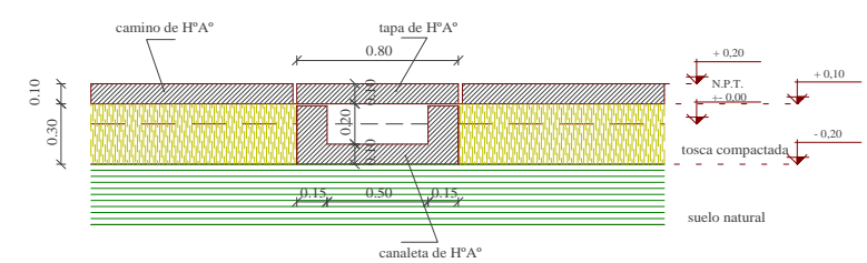
DETALLE SECTOR 1
