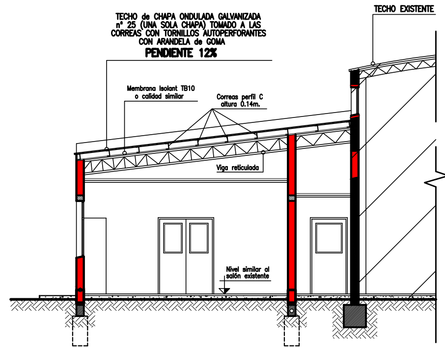
CORTE A-A'
