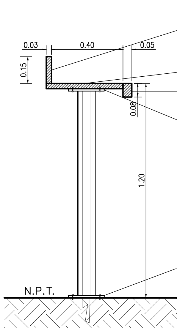
Corte detalle 1-1'
