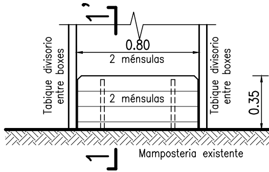
Planta asiento 9
