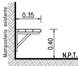
Corte 1-1'
