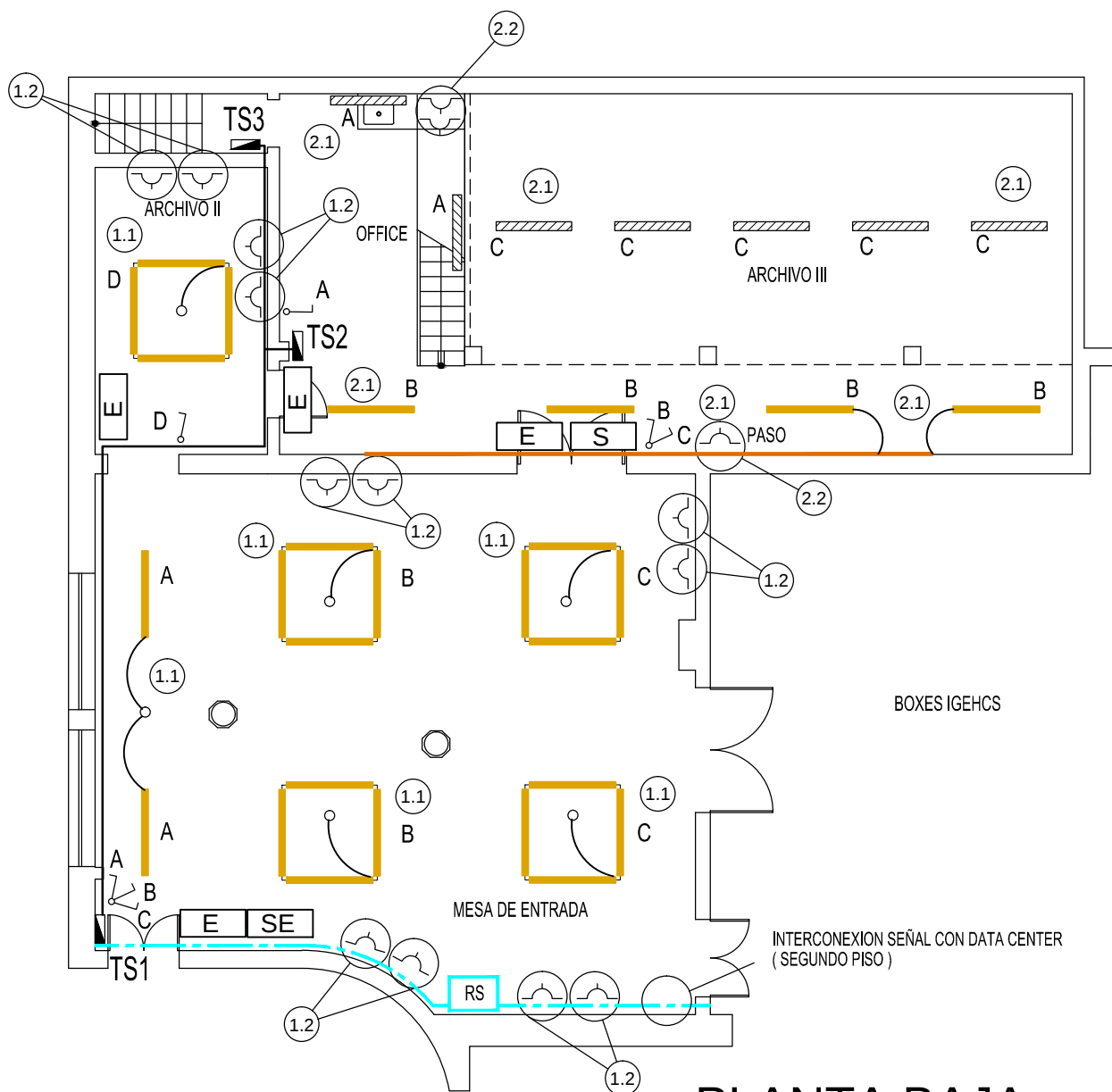
PLANTA BAJA
