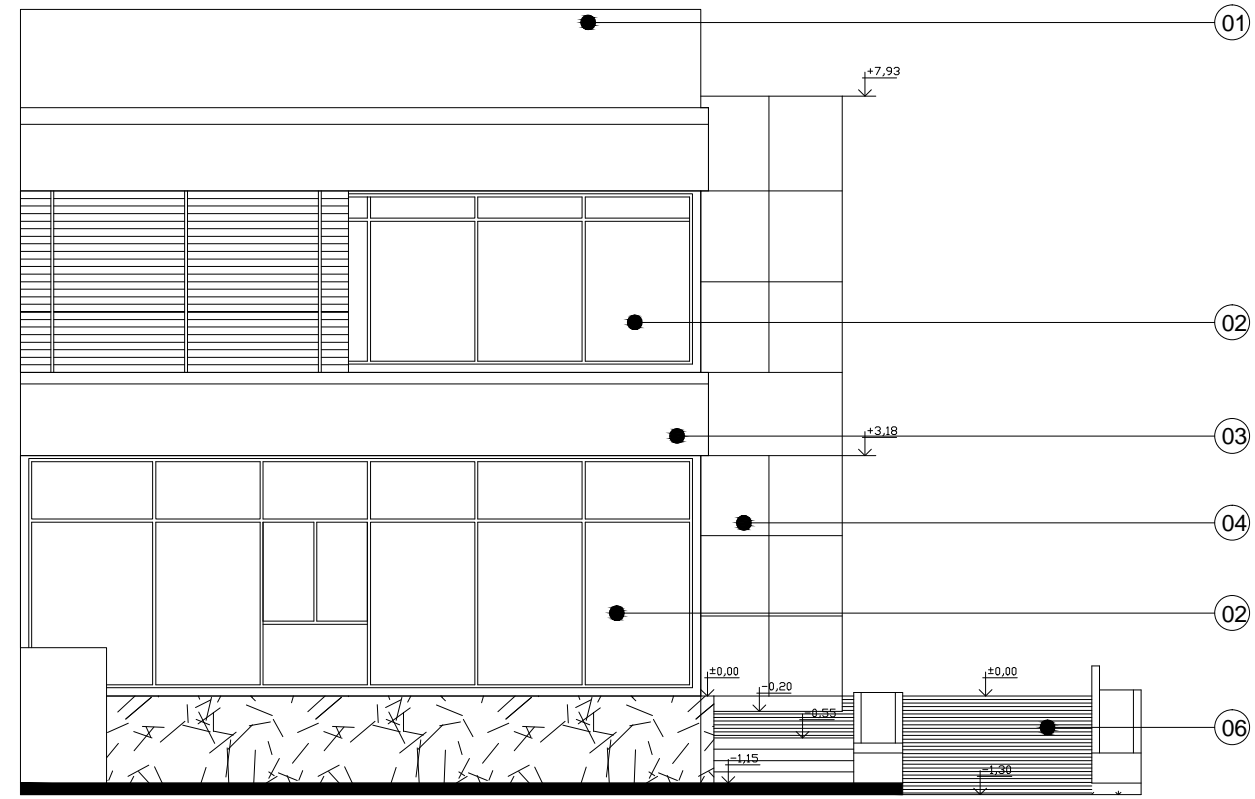
VISTA LATERAL
